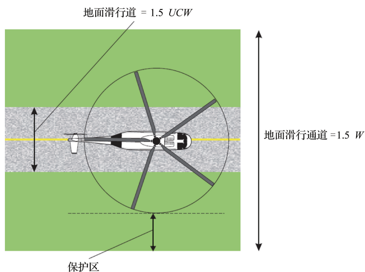
图 4.1.6 地面滑行道和地面滑行通道
