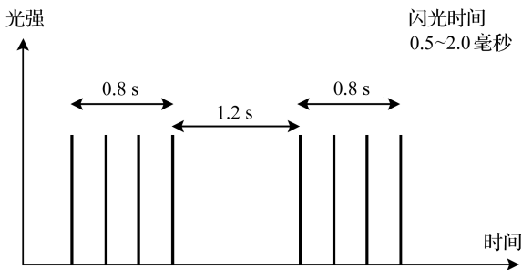
图 6.3.2-1 直升机场灯标闪光特性
