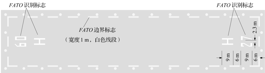
图 6.2.5-2 跑道型 FATO 识别标志（TLOF 与 FATO 重合）
