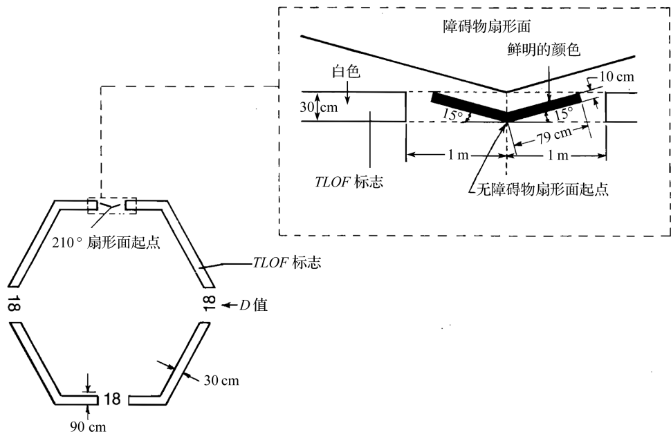
图 6.2.11 直升机水上平台无障碍物扇形面标志
