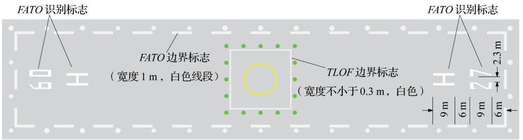
图 6.2.5-1 跑道型 FATO 识别标志（TLOF 与 FATO 不重合）
