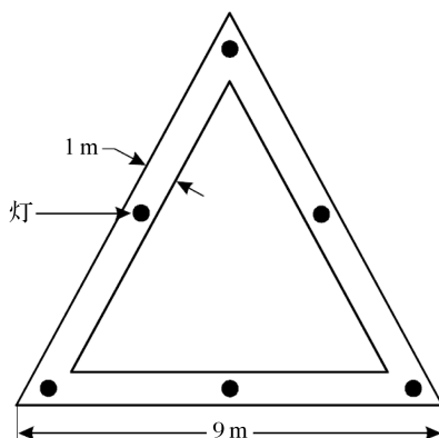
图 6.2.7 瞄准点标志
