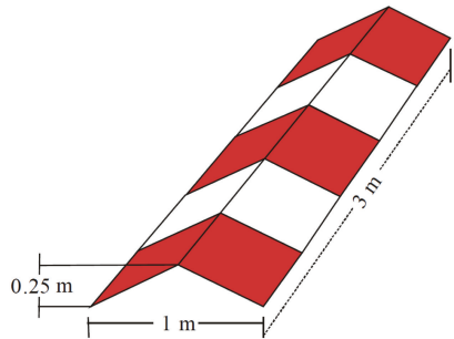
图 6.2.4-1 表面直升机场 FATO 边界标志物（仅示意红白相间情况）
