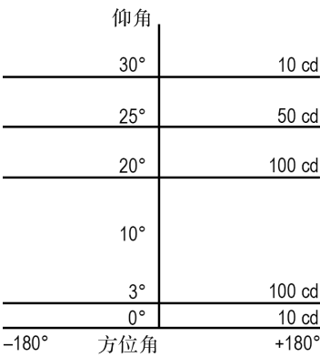
图 6.3.7 FATO 边界灯和瞄准点灯的光强分布
