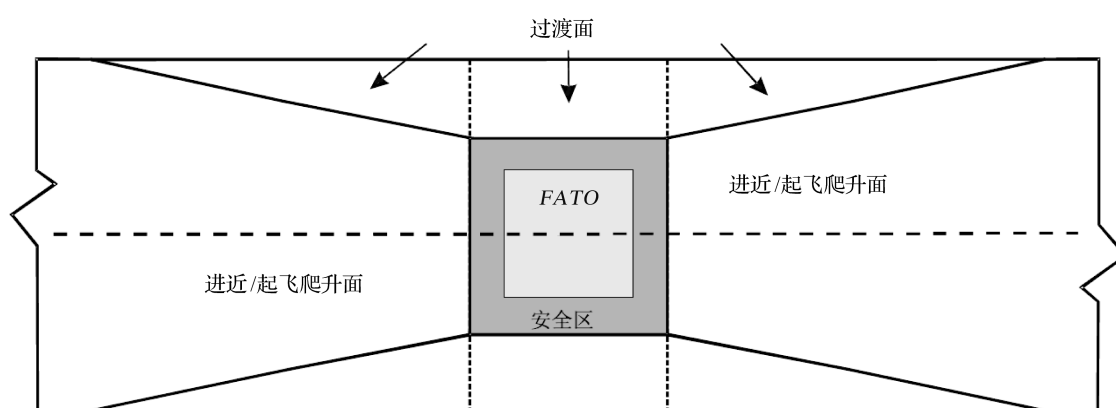
图 5.2.1-8 过渡面
