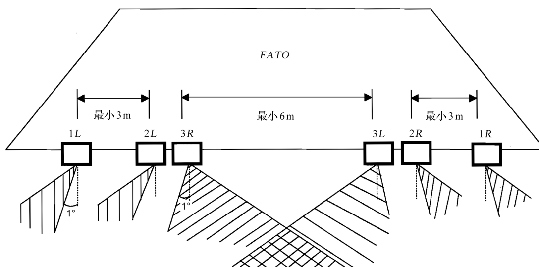
图 6.3.5-1 目视定向引导系统：灯具布置示意
