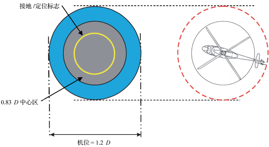
图 4.1.8-1 直升机机位
