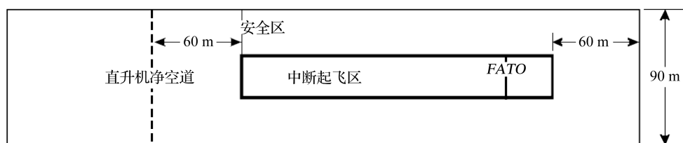
图 4.1.5-2 仪表 FATO 的安全区
