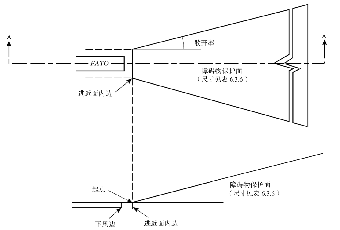
图 6.3.6-3 目视进近坡度指示系统的障碍物保护面
