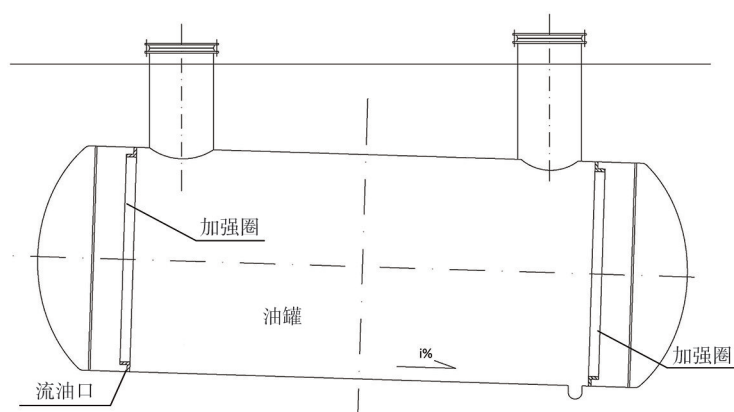
图 6.4.2-1 卧式油罐内的贯通形式
