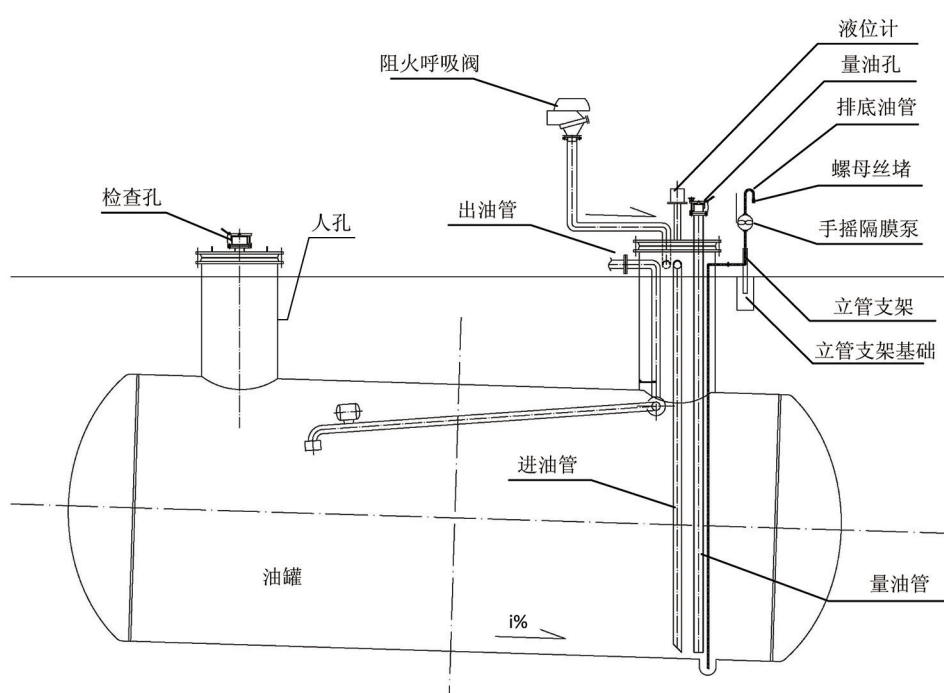
图 6.1.4-2 某机场埋地油罐工艺
