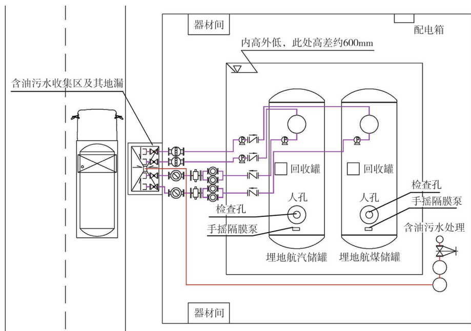
图 8.3.1-2 某机场油库综合管线图
