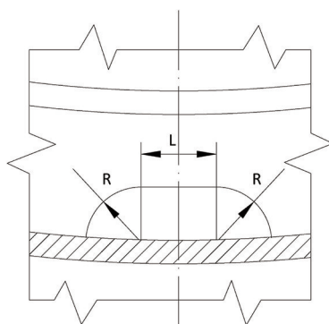
图 6.4.2-2 加强圈贯通形式——加强圈流油口示意图
