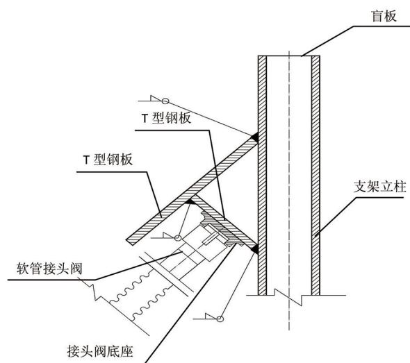
图 6.5.8-1 T 型支架
