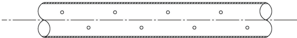
图 6.3.5-2 渗漏检查管开孔示意图
