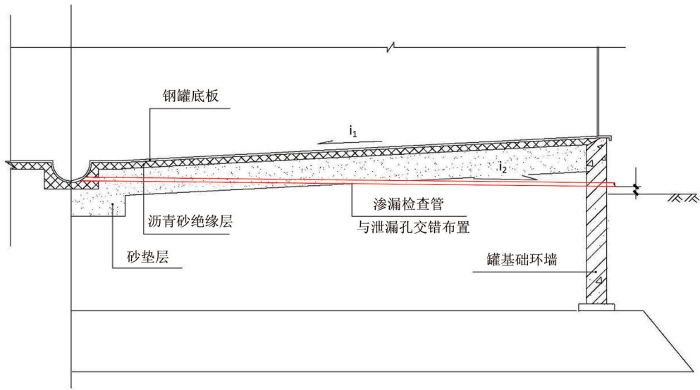
图 6.3.5-1 渗漏检查管与泄露孔布置
