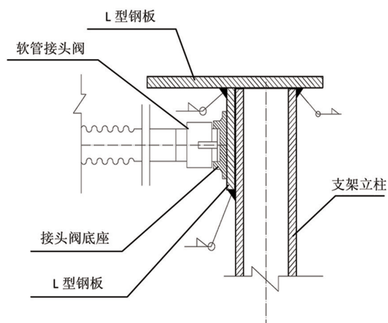
图 6.5.8-2 L 型支架
