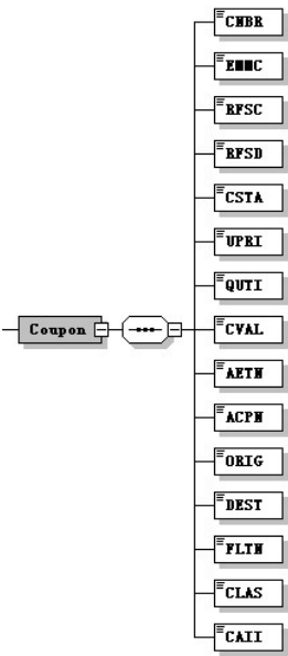
图30 查询响应报文结构图 5
