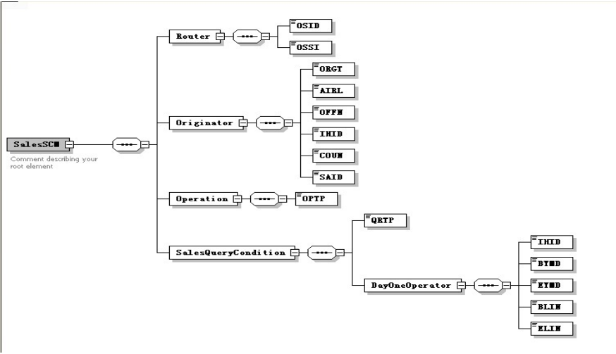
图33 销售统计请求报文结构图
