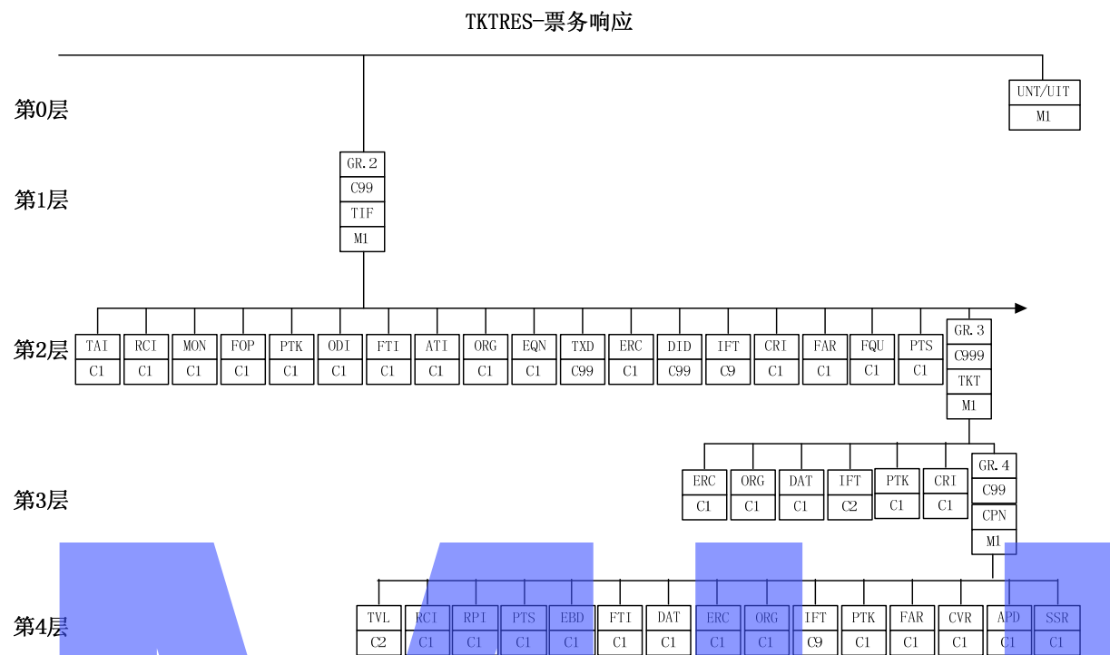
图17 TKTRES 报文分支图 2
