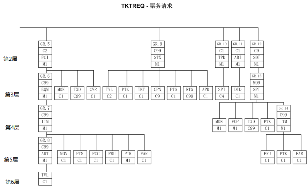
图14 TKTREQ 报文分支图 3
