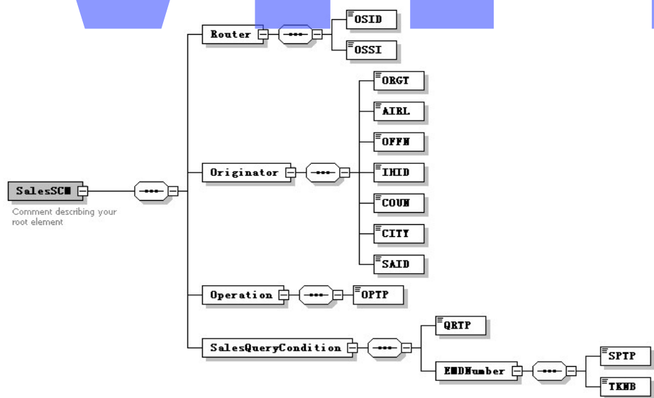
图25 查询请求报文结构图
