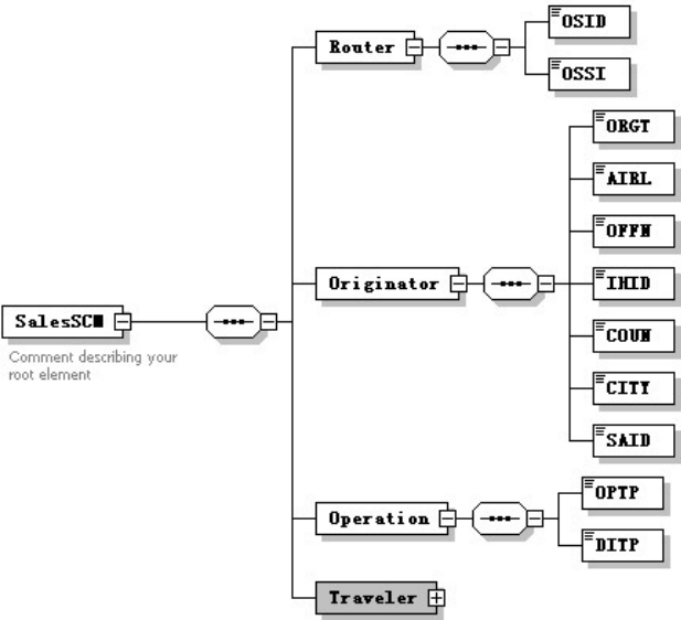
图20 出票请求报文结构图 1
