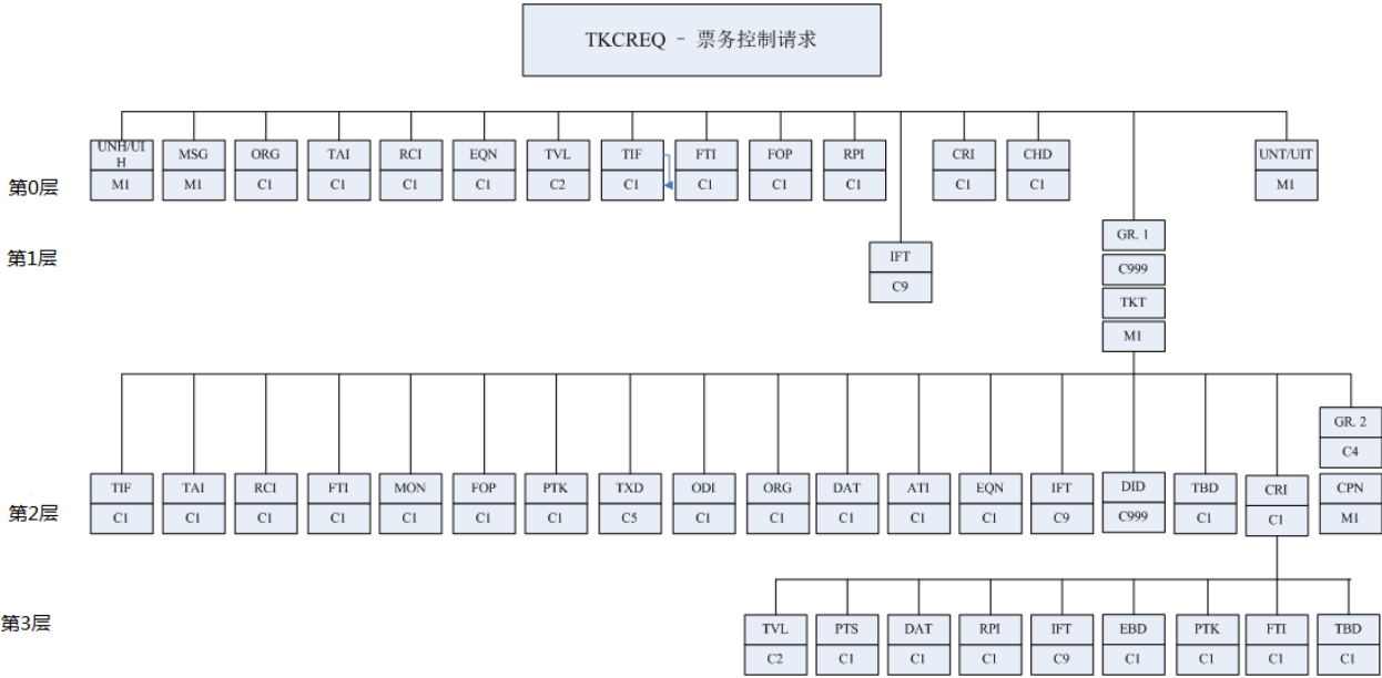
图5 TKCREQ 报文分支图
