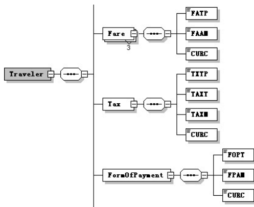
图22 出票请求报文结构图 3
