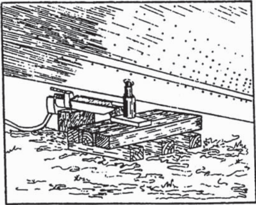
图 C.9 在软地上供千斤顶及气动起重袋用的基座
