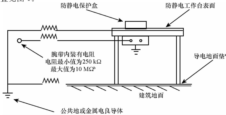
a 导电地面垫的尺寸应使工作人员在工作台处站着或坐着工作时能和它保持接地。 b 若工作电压是 240 V,要保证电流低于 1 mA,则腕带与导电垫接地心线之间的串联电阻值可由公式(1)计算。
