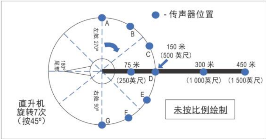
图S. 3 混合线性半圆阵列：7 个 45°旋转
