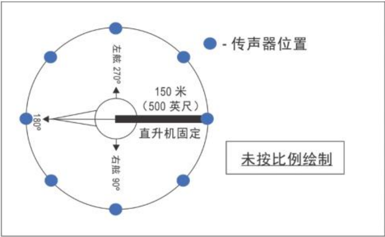
图S. 2 圆形传声器阵列
