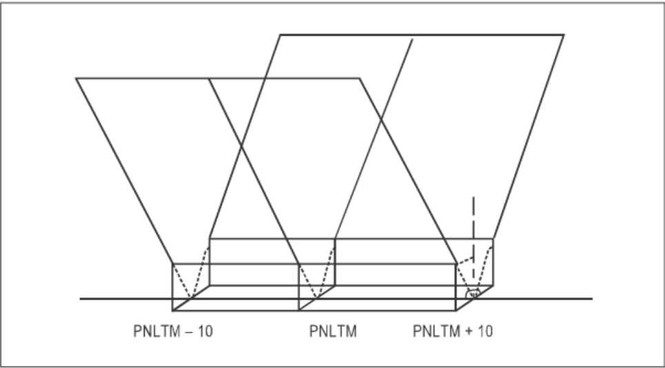
图H.1 直升机横向偏离容差
